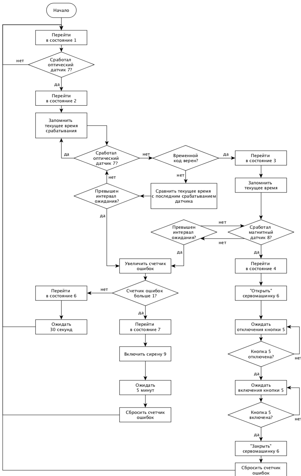
Рис. 5 – алгоритм работы программной части системы
