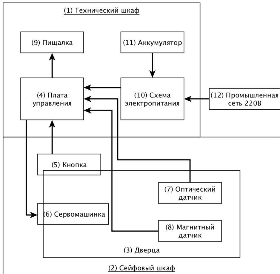
Рис. 3 — структурная схема мехатронного устройства
