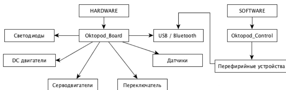
Рис. 10 – Структурное описание устройства Oktopod Studio
