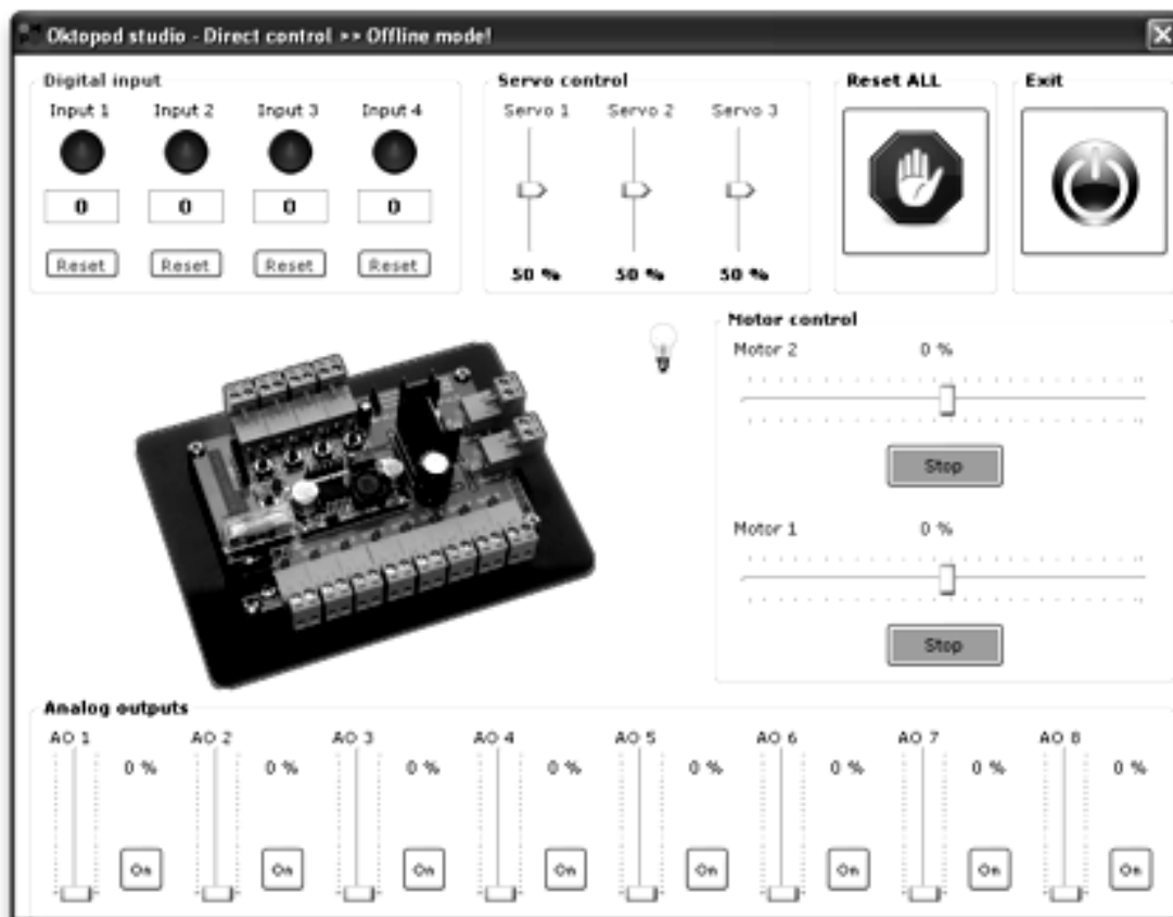
Рисунок 12 – Окно управления и мониторинга Oktopod_Control
