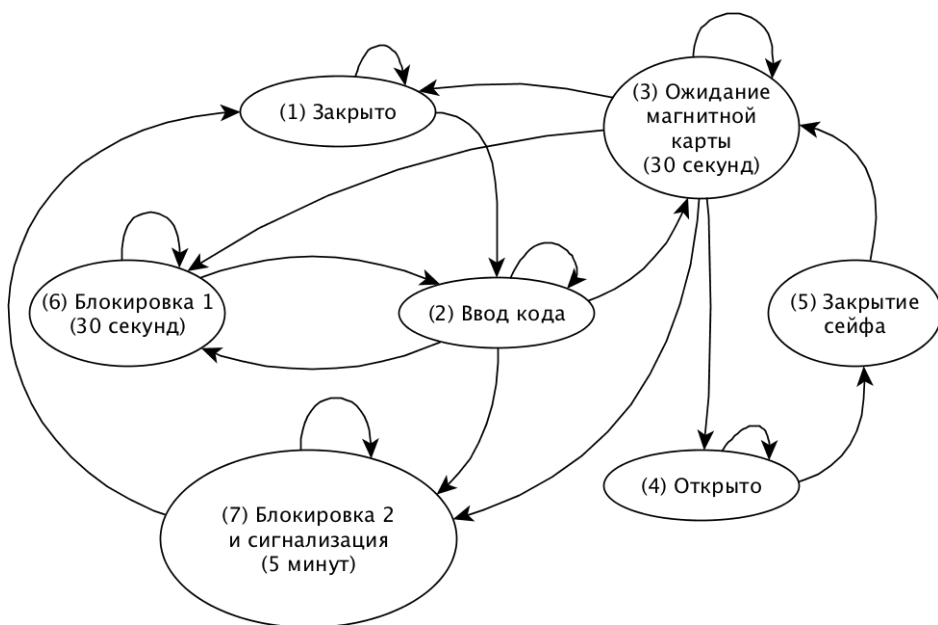
Рис. 4 – машина состояний мехатронного устройства сейфа
