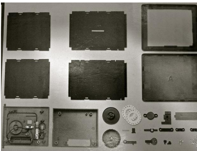
Рис.2 – состав деталей исходного прототипа
